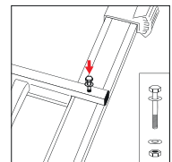
3) Brechen Sie das dünne Kunststoffteil, um den Stabilisator zu befestigen
